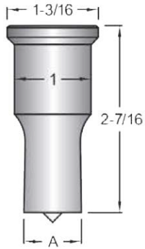
740 Punch
